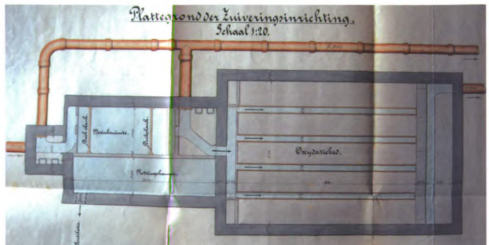
Plattegrond van de zuiveringsinstallatie.
